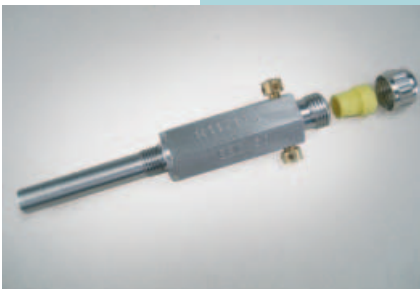
Abb. 2: Neue Fühlertasche EBL50/67 mit Kabelverschraubung
